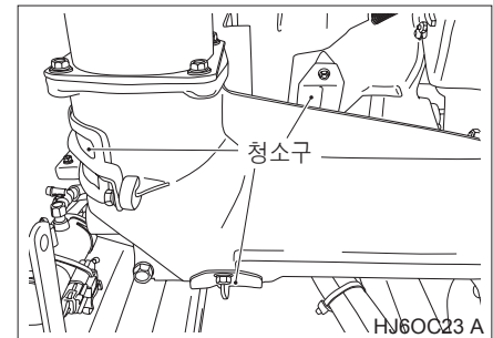
<1번메탈·2번 메탈 청소구>
