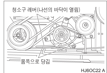
<1번 나선·2번 나선청소구>
