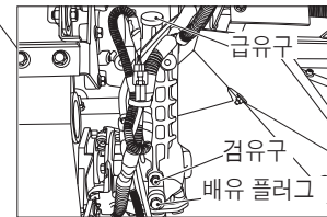
<인기 싱크로 기어케이스>
