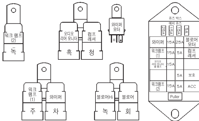
캐빈류 릴레이, 퓨즈 배치도
