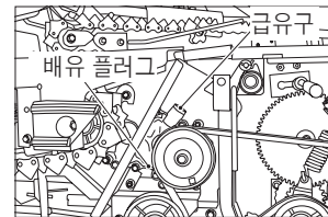
<배진팬 구동 기어케이스>
