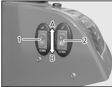
(1) 수평제어 (2) 유압 승강 실린더 (A) 상승 (B) 하강
