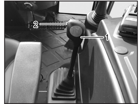
(1) 주변속 레버 (2) DE-clutch 버튼
