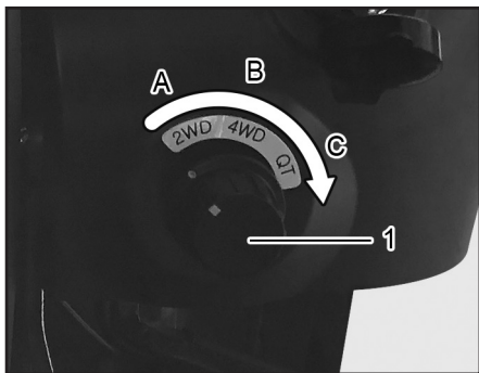
(1) 4륜구동/배속 스위치
