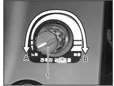
(1) 전후진 감도조절 스위치
