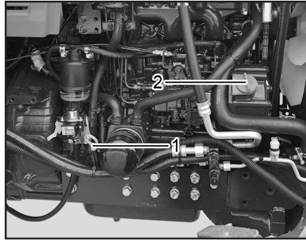
(1) 오일 게이지 (2) 오일 주입구
