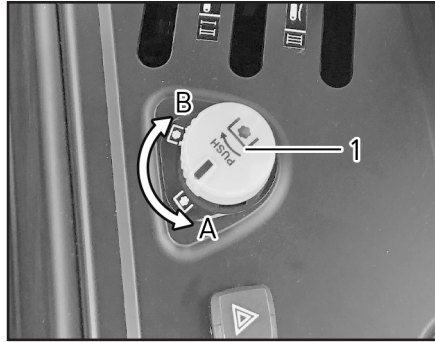
(1) PTO 절환 스위치 (A) OFF (B) ON
