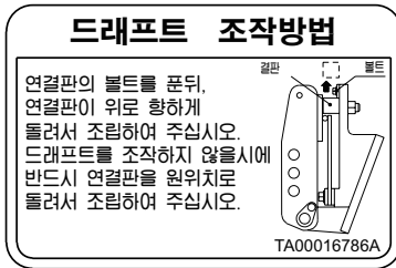
(12) 부품번호: TA00016786A
