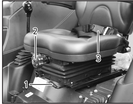
(1) 의자 전후조정 레버 (2) 쿠션 강약조정 노브 (3) 안전벨트
