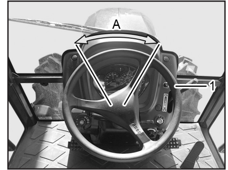
(1) 핸들 (A) 핸들 유격
