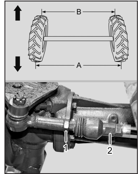
(1) 고정너트
