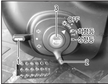
(1) 방향 지시 스위치 (2) 라이트 스위치 (3) 혼 버튼
