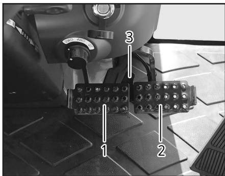
(1) 브레이크 페달 (좌) (2) 브레이크 페달 (우) (3) 연결 브라켓
